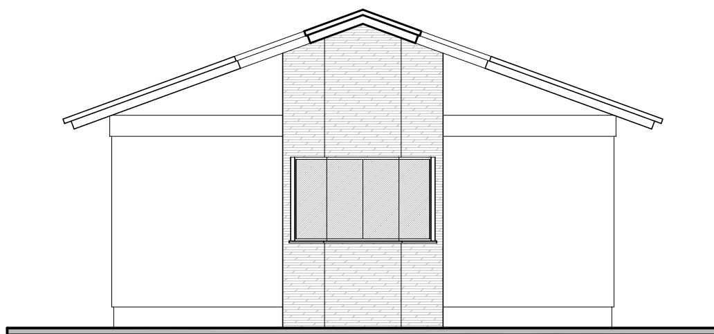
ELEVAÇÃO FRONTAL ESC. 1/75
