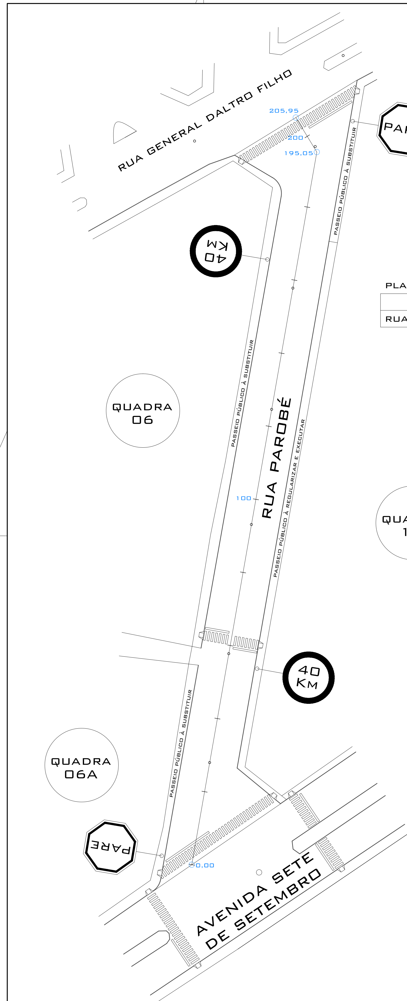
PROJETO DE SINALIZAÇÃO ESCALA- 1/500
